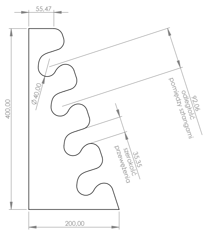
Uchwyt na Sztangi
